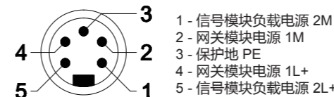
电源入 针端
