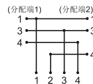
标准品电路图
