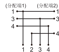
标准品电路图
