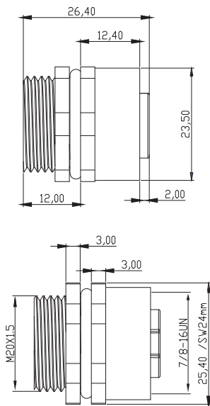
后板安装产品
