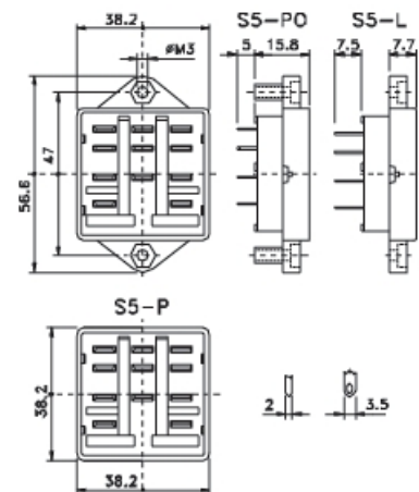
尺寸图解 [mm]
