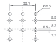
尺寸图解 [mm]
