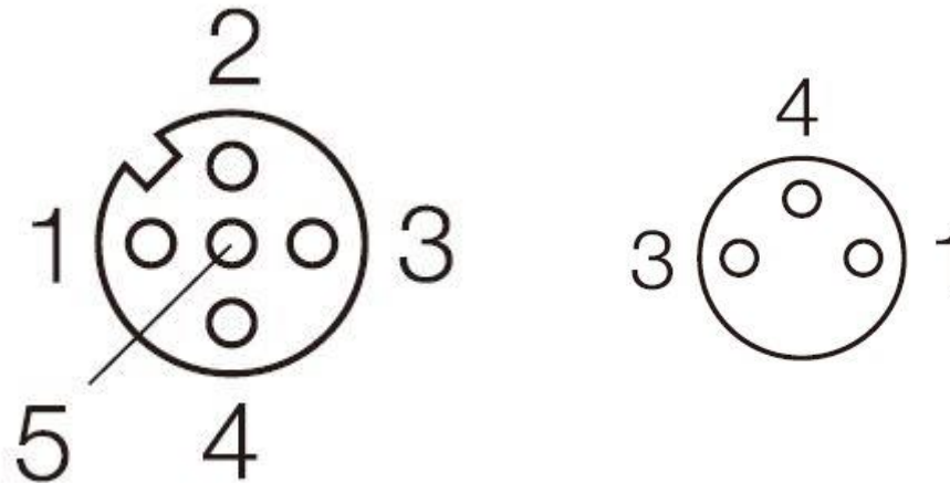
M12 接插件
